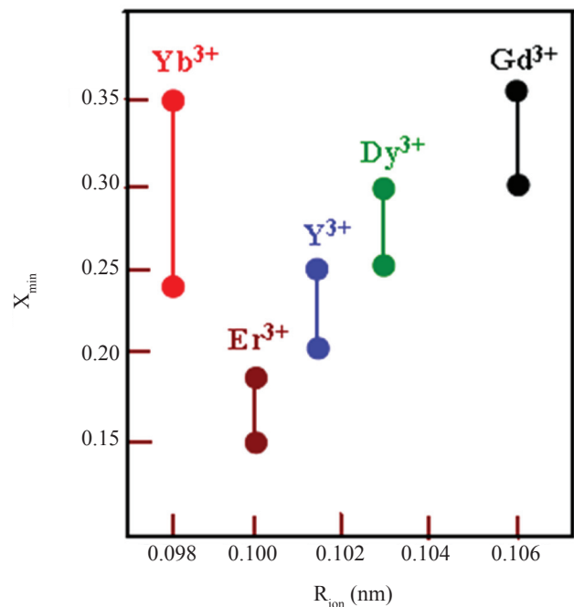
RAJAH 4. Julat kepekatan minimum, X_{\min} bahan dop yang diperlukan untuk menstabilkan fasa kiub fluorit dalam struktur (\text{Bi}_2\text{O}_3)_{1-x}(\text{Ln}_2\text{O}_3)_x melawan nilai jejari ion ( R_{\text{ion}} ) lantanid Verkerk & Burggraaf (1981)
