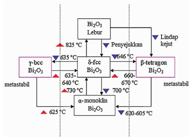
RAJAH 2. Peralihan fasa oksida bismut. Medernach & Snyder (1978)
